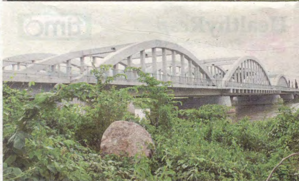
Jambatan Merdeka menggunakan reka bentuk asal iaitu tiga lengkung bagi kedua-dua jambatan yang dibina.
